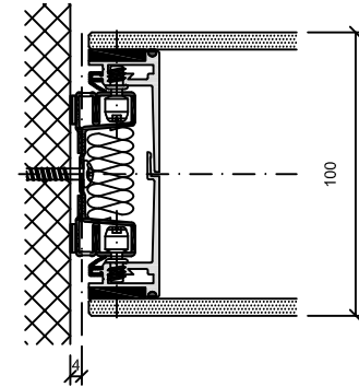
Wandanschluss
