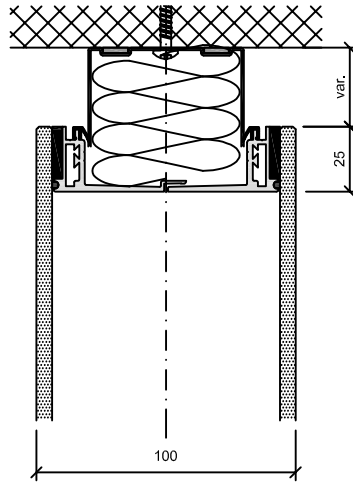
Deckenanschluss
