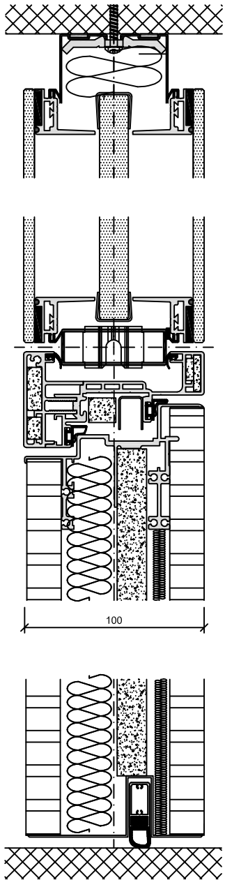
Vertikalschnitt
