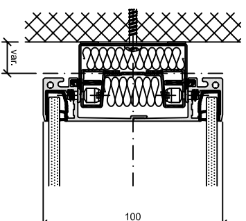
Anschluss variabel
