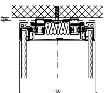
Wandanschluss
