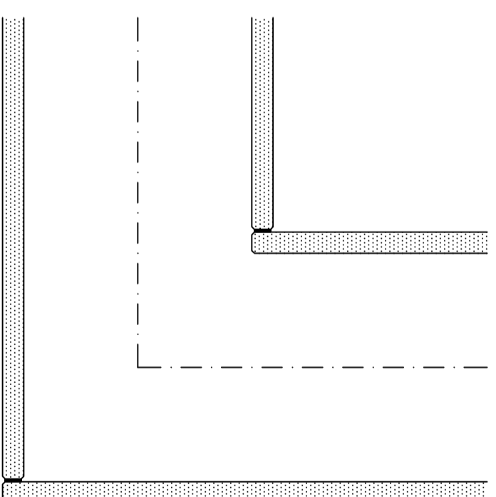
TTS - 90° - Ecke - stumpf Horizontalschnitt 1 : 2
