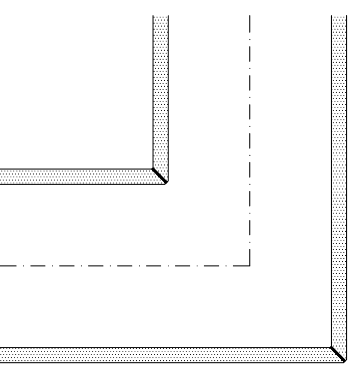
Elementstoss Horizontalschnitt 1 : 2
