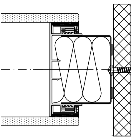
TTS Türe Vertikalschnitt 1:2
