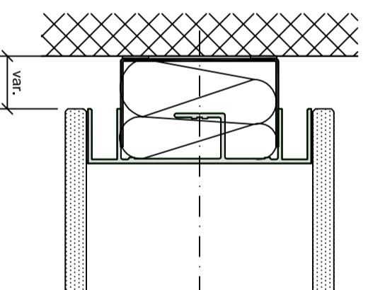
Wandanschluss Horizontalschnitt 1 : 2
