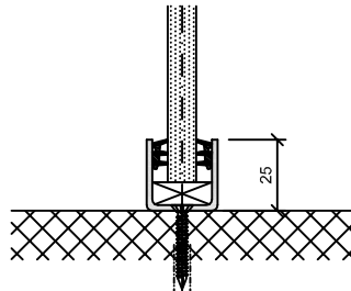
Bodenanschluss
