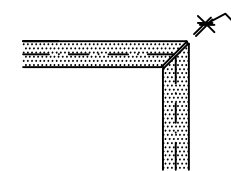
Ecke Gehrung
