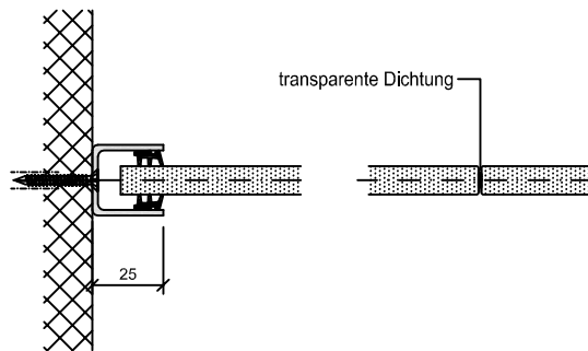
Wandanschluss und Elementstoss
