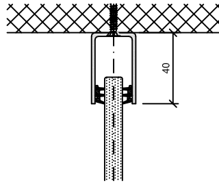
Deckenanschluss
