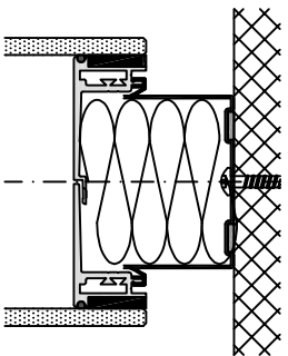
Vertikalschnitt
