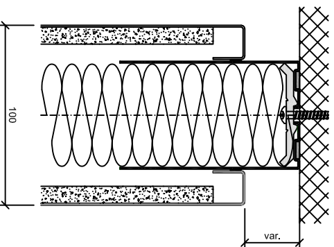
Deckenanschluss
