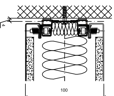
Wandanschluss
