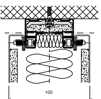
Anschluss variabel
