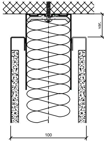
Deckenanschluss
