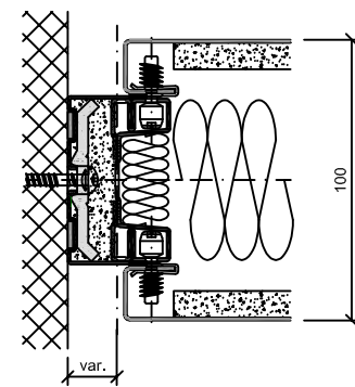
Anschluss variabel
