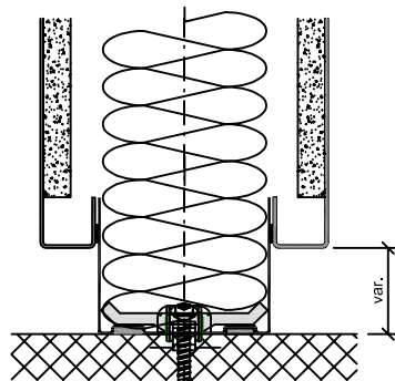
Bodenanschluss
