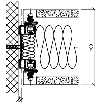
Wandanschluss
