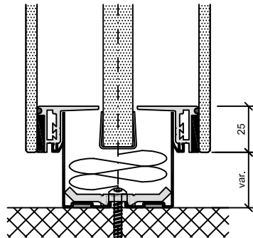
Bodenanschluss
