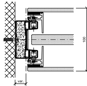
Anschluss variabel
