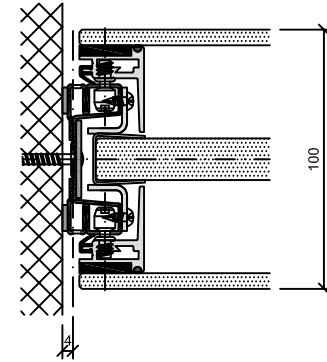
Wandanschluss
