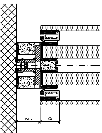
Bodenanschluss
