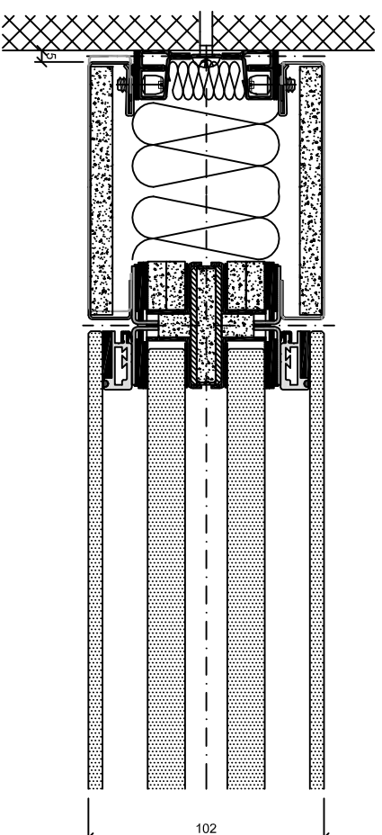
Wandanschluss
