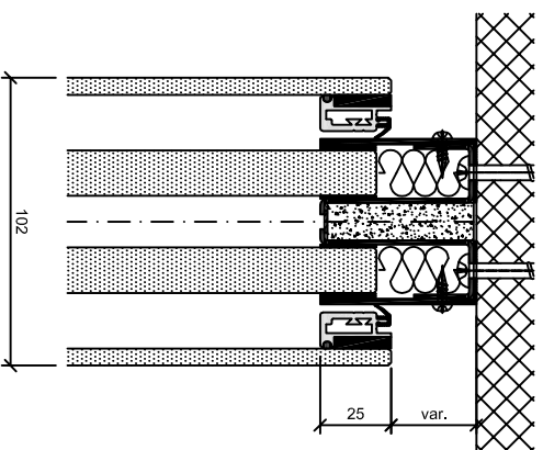
Deckenanschluss
