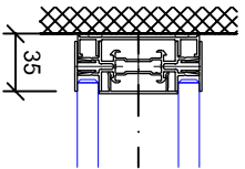
iQ-Structural 78 Wandanschluss Horizontalschnitt
